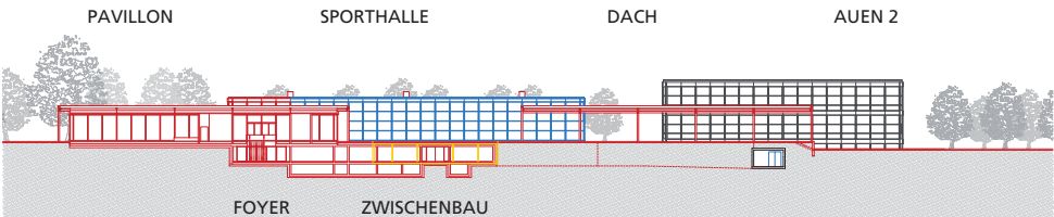
Ansicht Sporthalle/Auen 2
