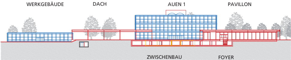
Ansicht Werkgebäude/Auen 1
